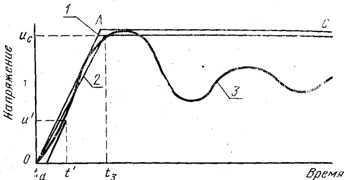
1—огибающая ПВН; 2—условная граничная линия ПВН; 3—собственное ПВН Черт. 5
