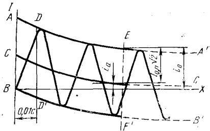
Периодическая и аperiodическая составляющие тока короткого замыкания
