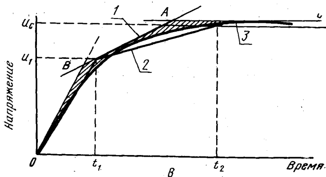
1—огибающая ПВН; 2—условная граничная линия ПВН; 3—собственное ПВН. Заштрихованные площадки приблизительно равны
