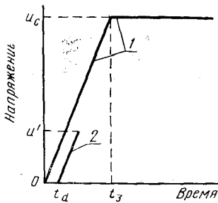
1—условная граничная линия ПВН; 2—линия запаздывания ПВН (параллельная граничной линии).
