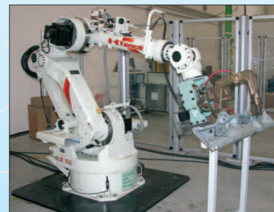
Spot welding using Servo Weld Gun Punktschweißen mit Servo Gun
