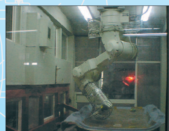
Water jet cutting Wasserstrahlschneiden
