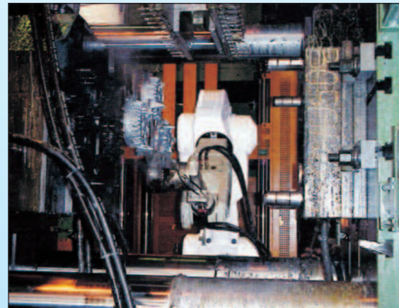
Die-casting Druckguß
