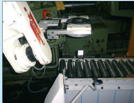
Loading & unloading Be- und Entladen
