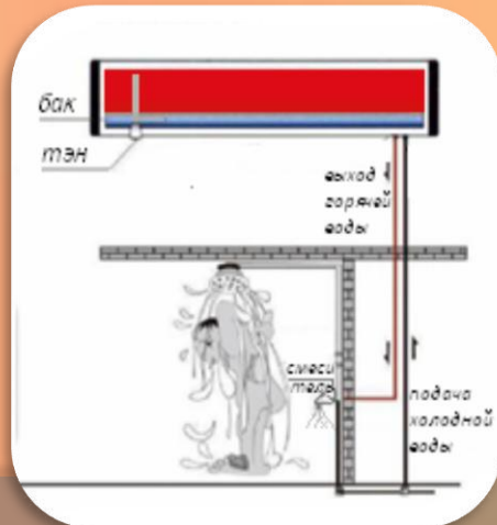
Схема солнечного водонагревателя без давления (термосифонная система)
