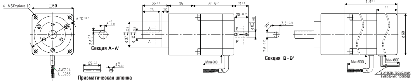
<Внешний вид двигателя со ступицей>
