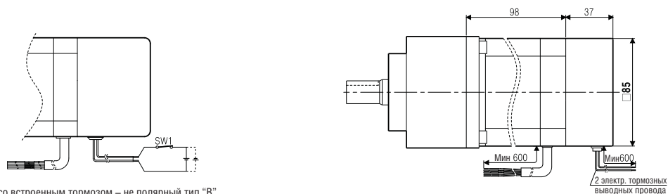
<Внешний вид двигателя со встроенным редуктором + тормоз>
