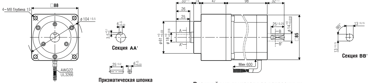
<Внешний вид двигателя со встроенным редуктором + тормоз>
