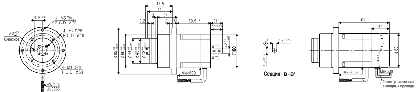
<Внешний вид двигателя со ступицей + тормоз>
