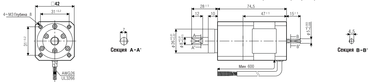
<Внешний вид двигателя со встроенным редуктором>
