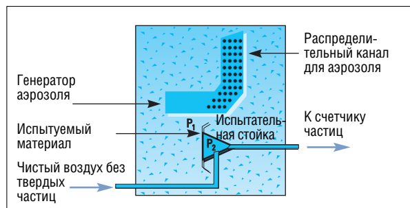
Рисунок 1. Испытательная камера
