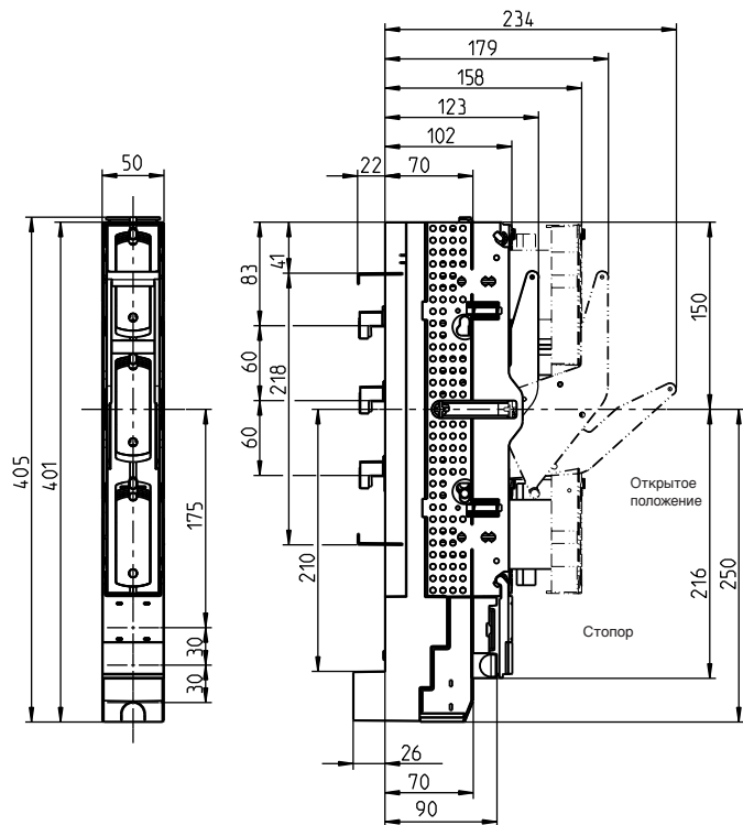
Вертикальные разъединители с предохранителем ЕЗ-НН, 00/100
