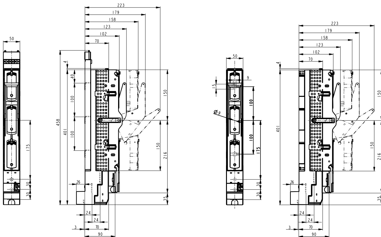
Вертикальные разъединители с предохранителем ЕЗ-НН, 00/100
