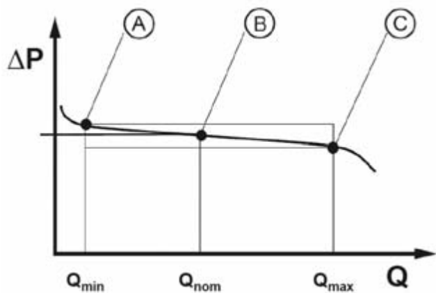
Рис. 6 Регулировочная характеристика
