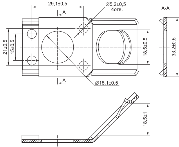
КАБ-200
