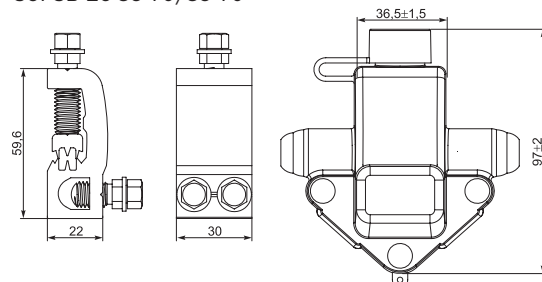
ЗОРЗБ-2С 35-70/35-70
