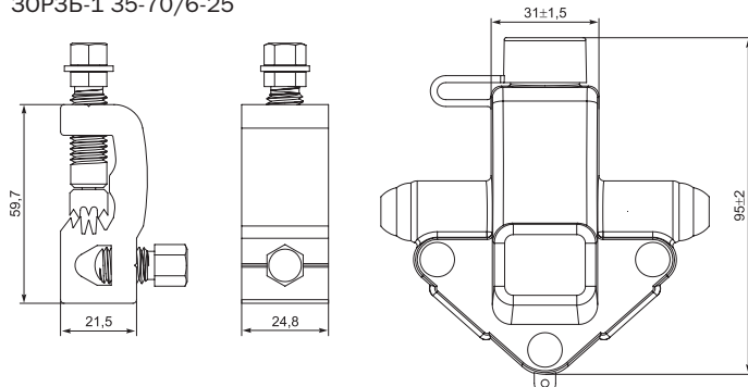
ЗОРЗБ-1 35-70/6-25
