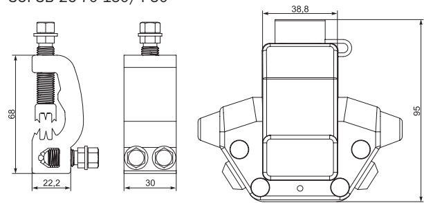
ЗОРЗБ-2С 70-150/4-50
