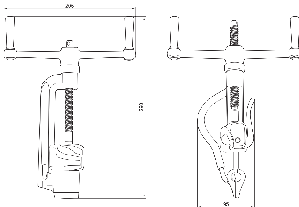
Инструмент ИНСЛ-1
