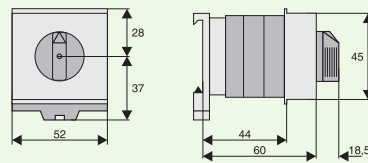
Размеры [мм]
