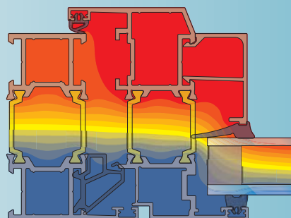
Sisään avattava ikkuna Inward opening window
