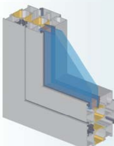
Sisään avattava ikkuna Inward opening window
