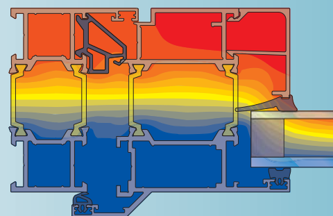
Ulos avattava ikkuna Outward opening window
