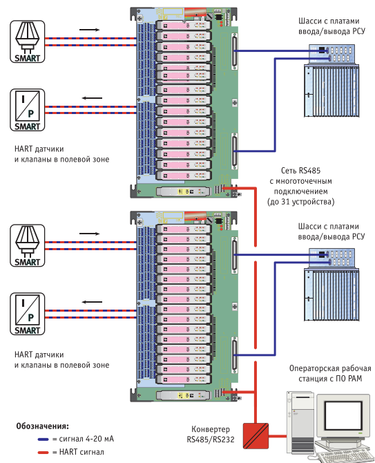
HiD 2000 плата с барьерами искробезопасности и HART мультиплексором
