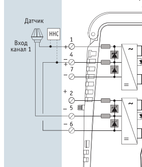
Включение HiD2030 с одним входом и двумя выходами
