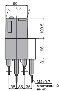
План крепежных отверстий (вид спереди)
