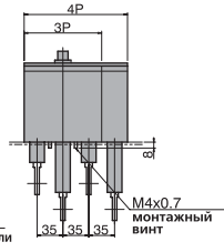
План крепежных отверстий (вид спереди)
