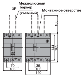
Переднее присоединение
