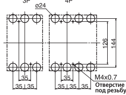
План крепежных отверстий (вид спереди)
