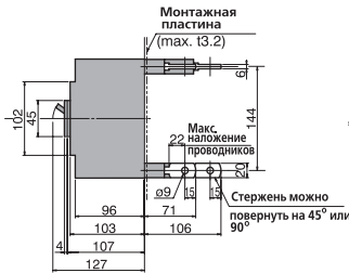
Заднее присоединение
