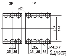
План крепежных отверстий (вид спереди)
