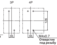
План крепежных отверстий (вид спереди)
