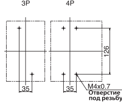
План крепежных отверстий (вид спереди)
