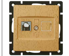
1xRJ45 40XX-051-9900
