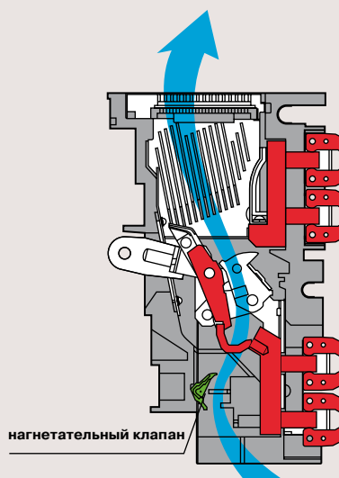
Поток воздуха проходит через нагнетательный клапан Защищено патентом
