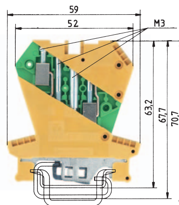
Закрытое исполнение
