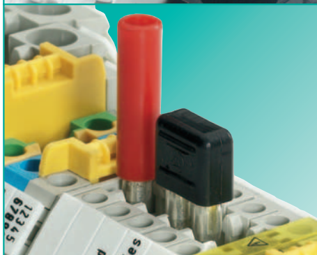
Штекерные гнезда Тестовые вставки Короткозамыкающие штекеры
