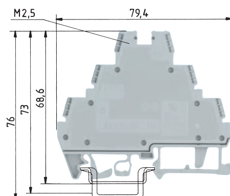
WK 2,5 - 3 D/U-NGN
