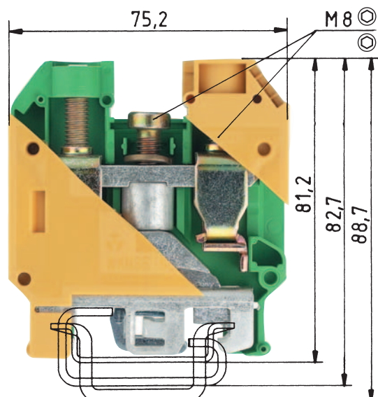
Закрытое исполнение
