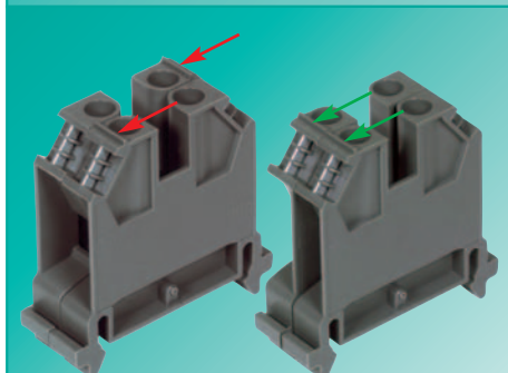
неправильный монтаж правильный монтаж
