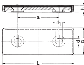
Маркировочные шильдики Поставляются в разобранном состоянии!
