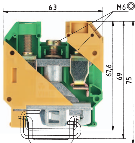
Закрытое исполнение
