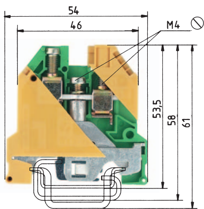
Закрытое исполнение
