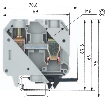
Закрытое исполнение
