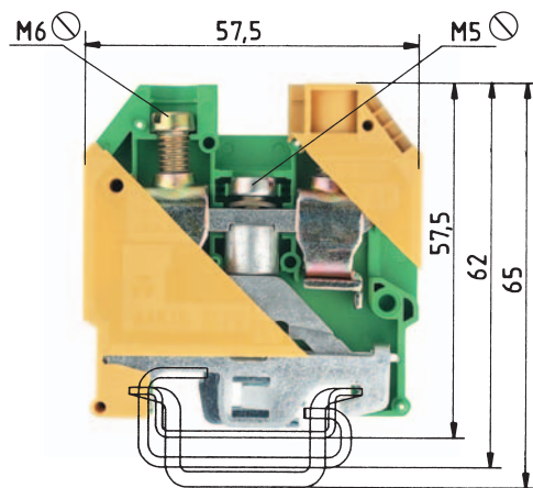
Закрытое исполнение
