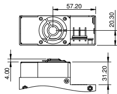
FAN OPTION
