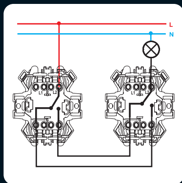
Выключатель проходной/переключатель
