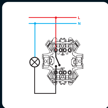
Выключатель однополюсный
