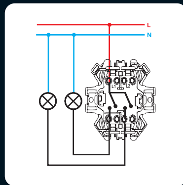
Двухклавишный выключатель
