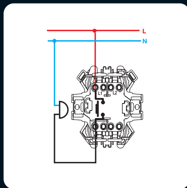
Клавишная кнопка
