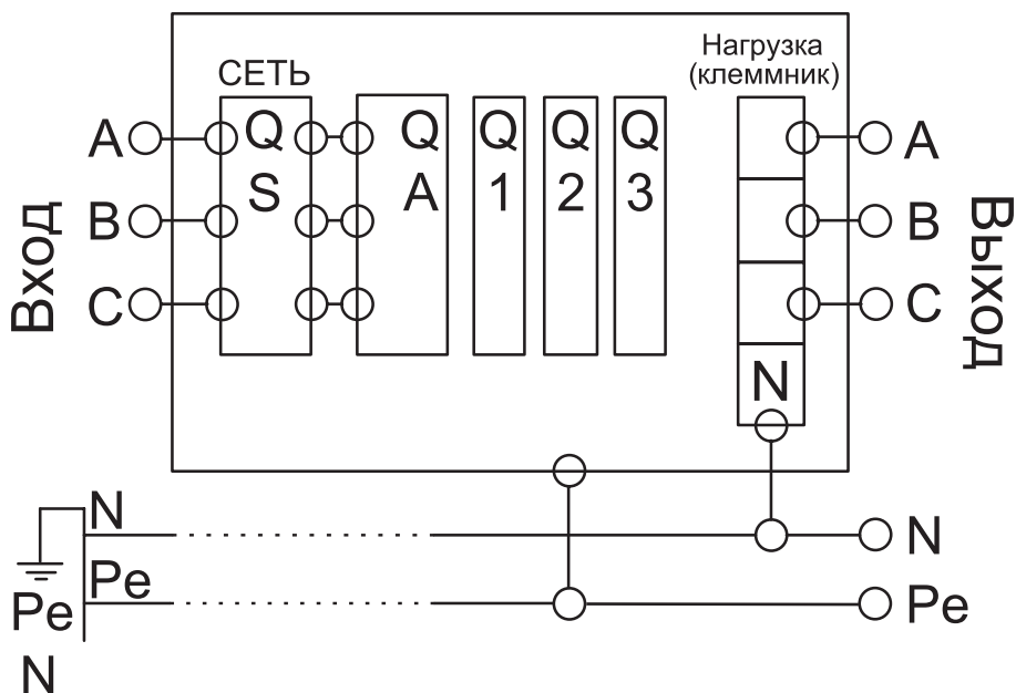
Рис.1 Схема подключения
