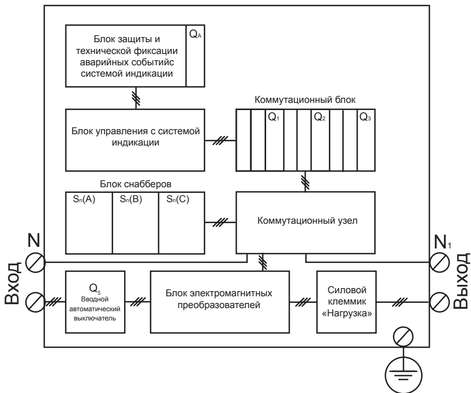
Рис.2 Блок-схема нормализатора
