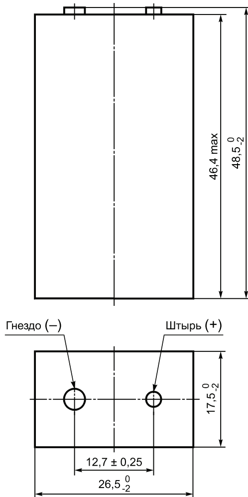
Рисунок 20 — Размеры батарей 6F22, 6LR61
