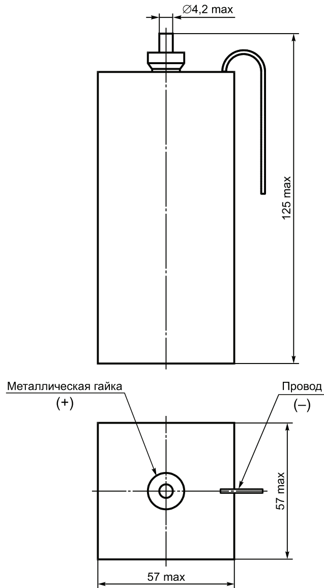
Рисунок 9 — Размеры батареи S4
