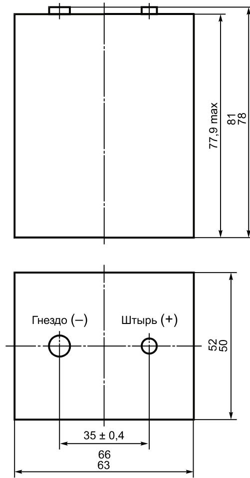
Рисунок 21 — Размеры батареи 6F100
