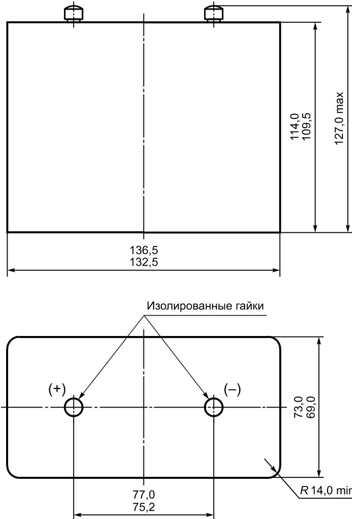
Рисунок 17 — Размеры батарей 4R25-2, 4LR25-2
