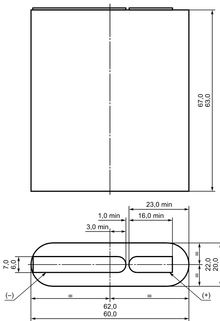
Рисунок 10 — Размеры батарей 3R12C, 3R12P, 3R12S, 3LR12
