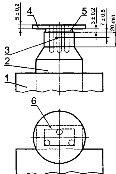
1 – нагревательный элемент; 2 – металлическая часть; 3 – термопара; 4 – изоляционная плита; 5 – прокладка; 6 – контур вилки
