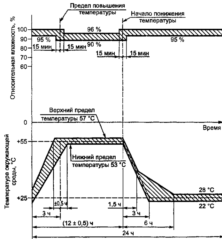
Рисунок 22 – Цикл испытания на надежность (9.22.1.3)
