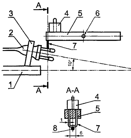
Рисунок 12 – Установка для испытания на сжатие
