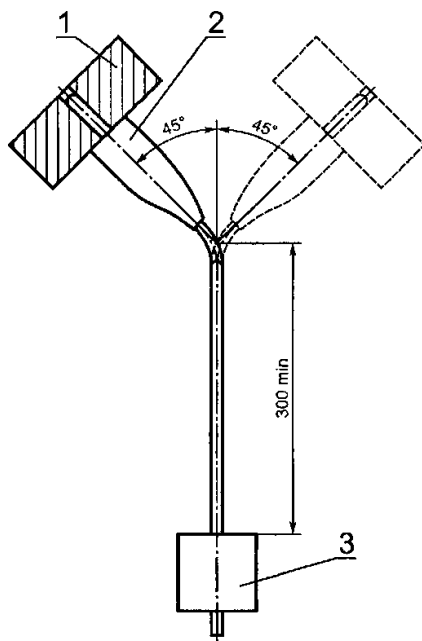
1 – устройство для закрепления образца; 2 – образец; 3 – груз
