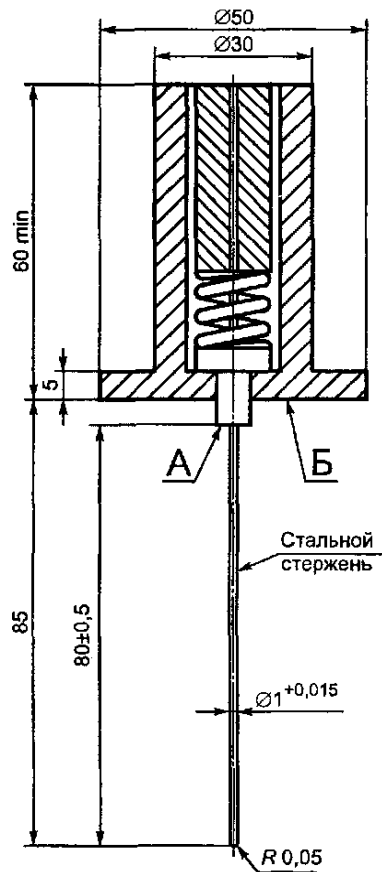
Рисунок 3 – Измерительный прибор для проверки недоступности токоведущих частей
