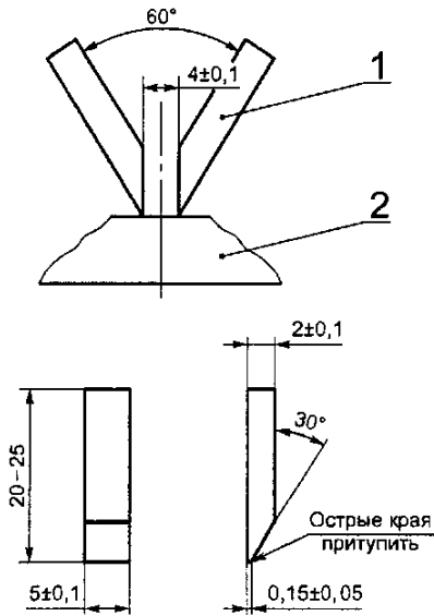
1 – электрод; 2 – образец
