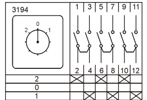
ПК16-12 С3194
