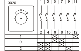
ПК 16-12 А3020
