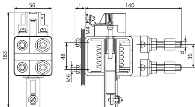
Реле РЭО-401 2ТД
