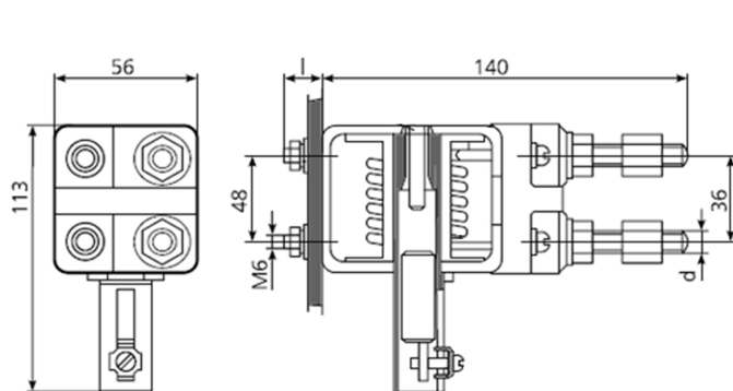
Реле РЭО-401 6ТД
