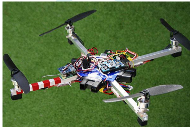
Робот-квадрокоптер на Arduino
