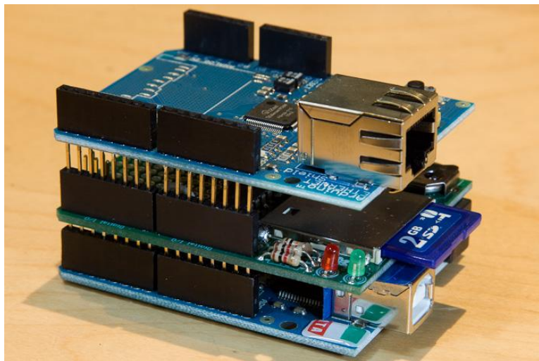
Web – сервер на Arduino
