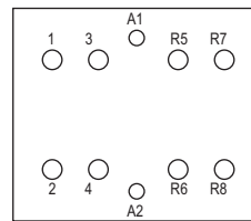
2НО + 2НЗ контакта
