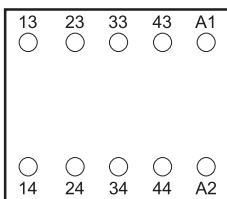
4НО контакта
