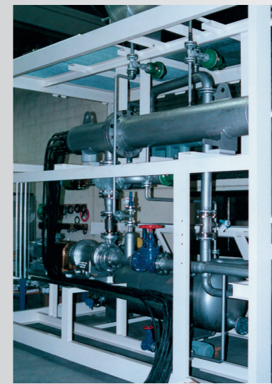
600 кВт, 400 В, 3 фазы Циркуляционные нагреватели оснащены ТНР элементами 17 x 35 кВт Жидкость: масляный теплоноситель, авиационная испытательная лаборатория
