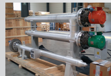
394 кВт для А-2301 и 110 кВт для А-2302, 400 В, 3 фазы Среда: углеводород + водород
