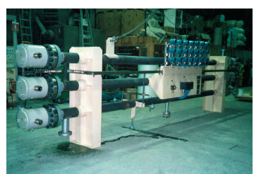
435 кВт, АТЕХ. Циркулирующая в нагревателе жидкость: Парафин при 325 °C
