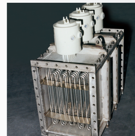
EExdIIC Электрический конвектор 3x 20 кВт Максимальное рабочее давление 1 бар
