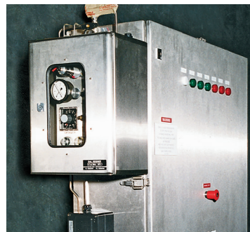
Контрольная коробка EXpII 70° С
