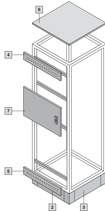
Комплектующие шкафа
