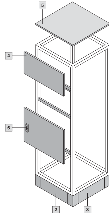
Комплектующие шкафа
