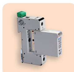
Съемный УЗИП Surge Trap®
