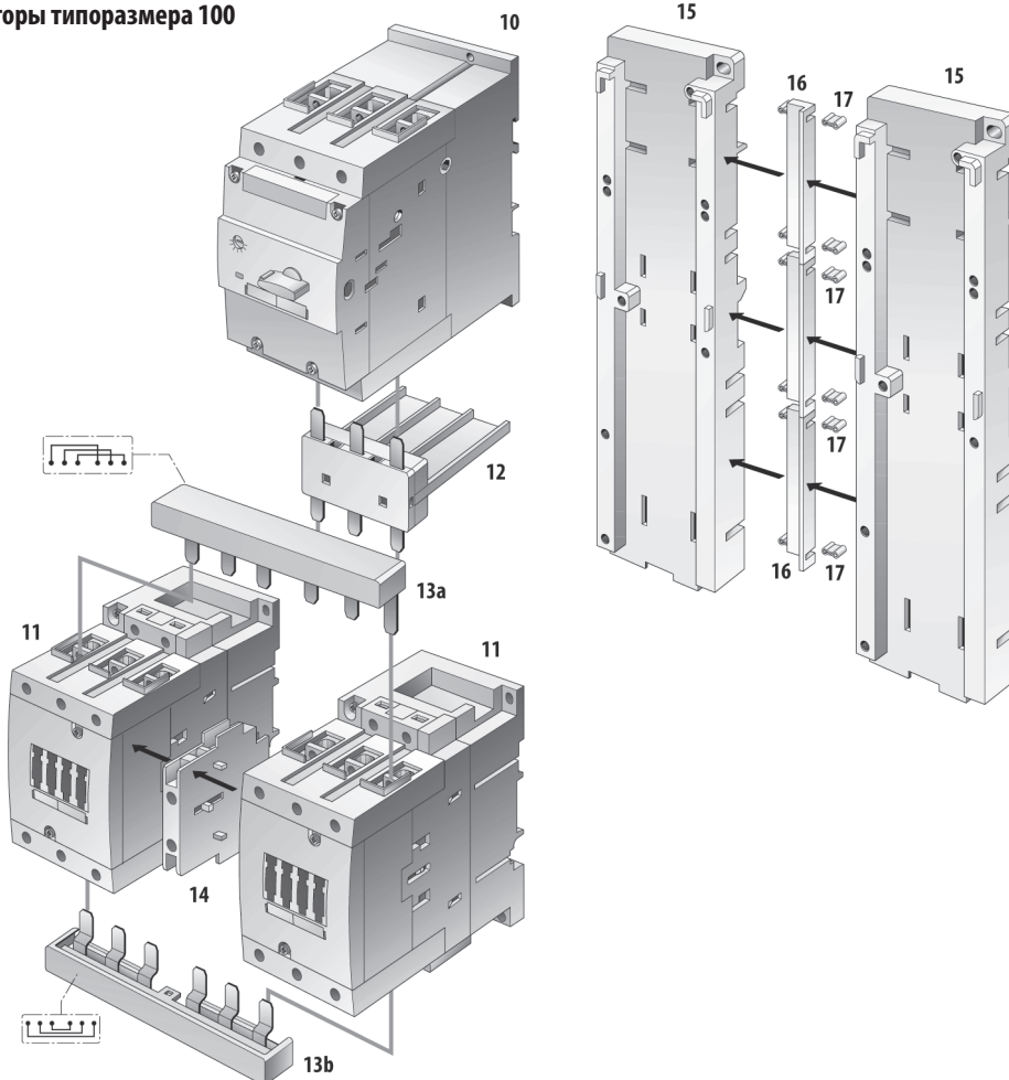
Автоматический выключатель защиты двигателя и контакторы типоразмера 100
