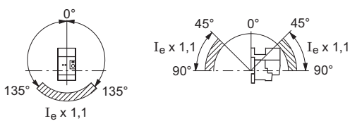
Реле защиты двигателя (с адаптером)
