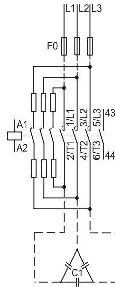
Контакты SC, типоразмер 25 и 100
