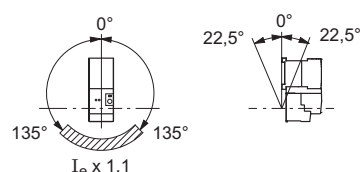
Реле защиты двигателя и контактор
