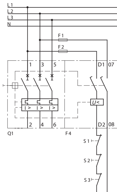
Пример подключения кнопки „STOP“
