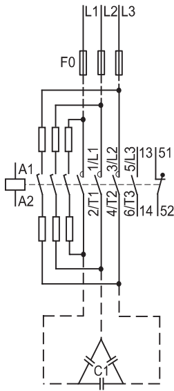
Контакты SC, типоразмер 12
