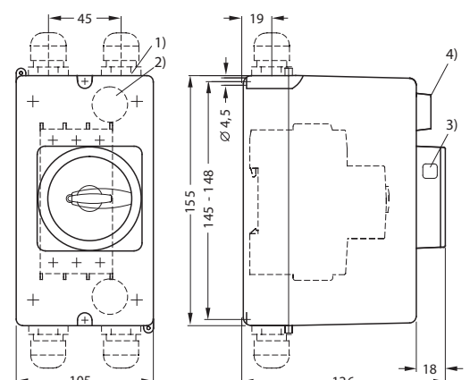
Изоляционный кожух OD-SM253-K52, OD-SM253-K53
