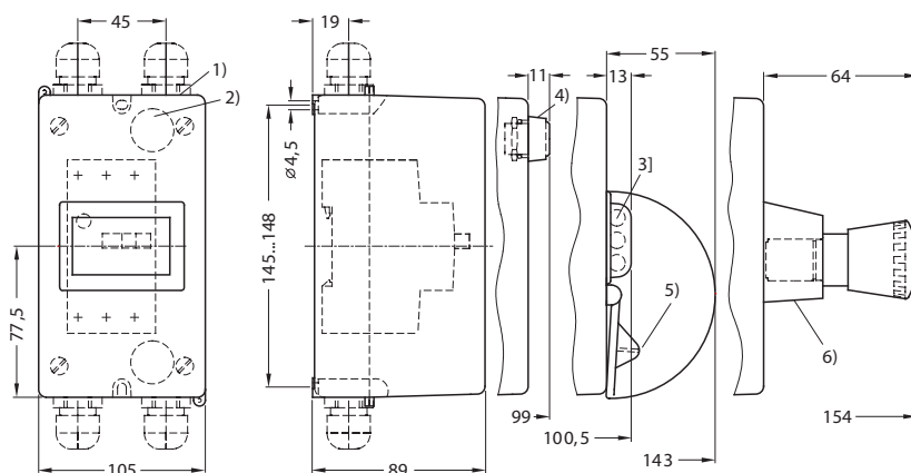
Изоляционный кожух OD-SM123-K51
