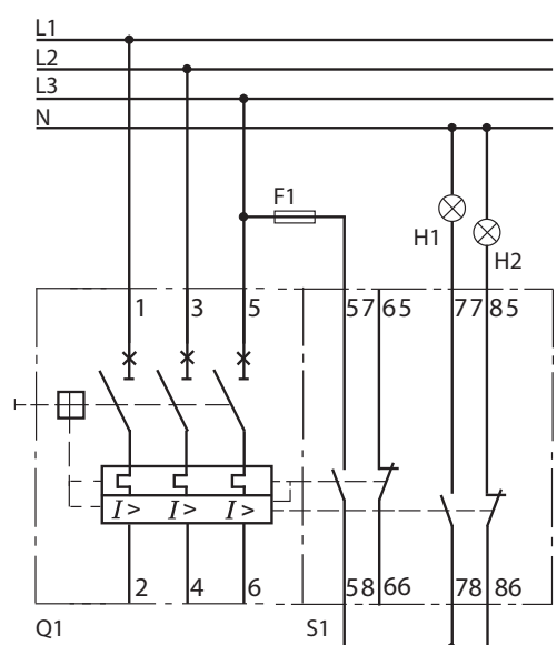
Пример подключения сигнального выключателя
