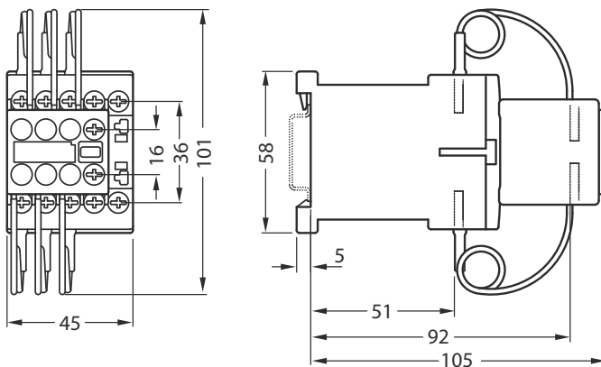
Контакты SC, типоразмер 12
