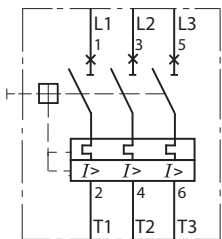
Авт. выключатель защиты двигателя
