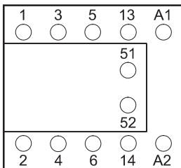
Контакты SC, типоразмер 12
