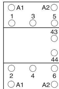
Контакты SC, типоразмер 25 и 100
