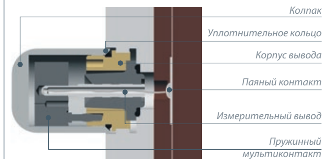
Рис. 11. Измерительный вывод с заземляющим мультиконтактом
