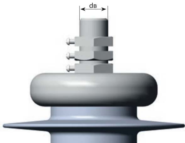
Рис. 23. Контактная шпилька ввода 35 кВ
