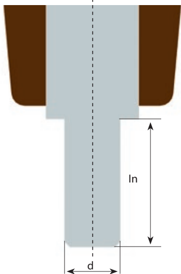
Рис. 21. Нижнее подсоединение вводов 35 кВ
