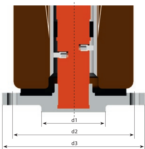
Рис. 22. Нижнее подсоединение вводов 110 и 220 кВ
