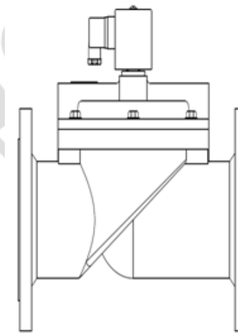
Рисунок 1. Устройство
