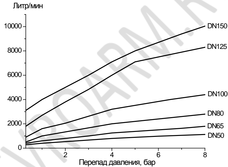
Диаграмма 1. Зависимость расхода от давления
