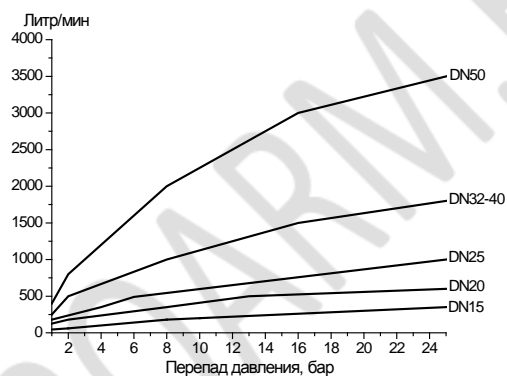
Диаграмма 1. Зависимость расхода от давления
