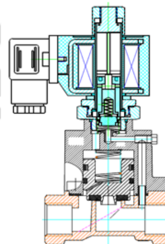
Рисунок 1. Устройство
