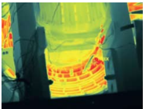
Теплограмма трансформатора ТРСЭП-12500/10
