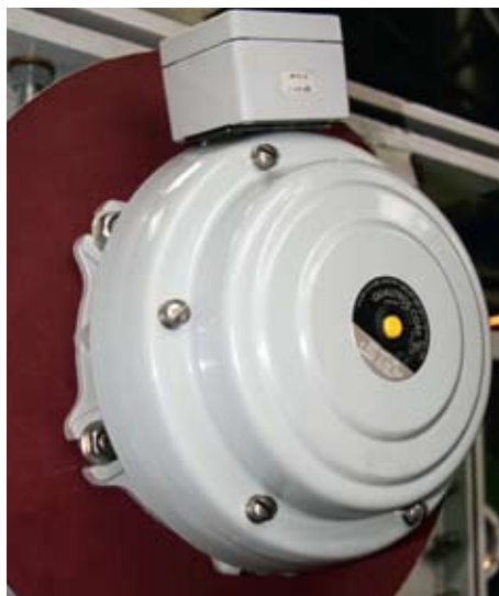
Предохранительный клапан фирмы «Qualitrol» (США)
