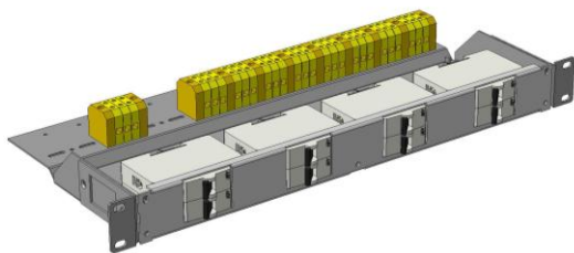
Модуль распределения Штиль MP-21-08
