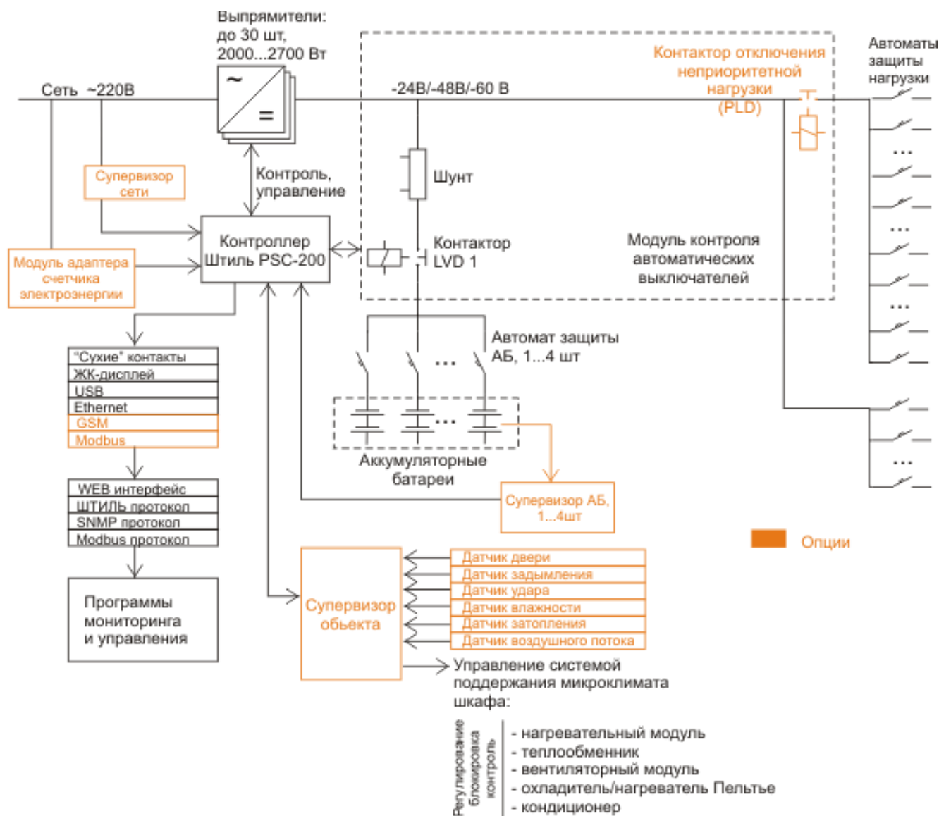
Функциональная схема установок питания постоянного тока Штиль
