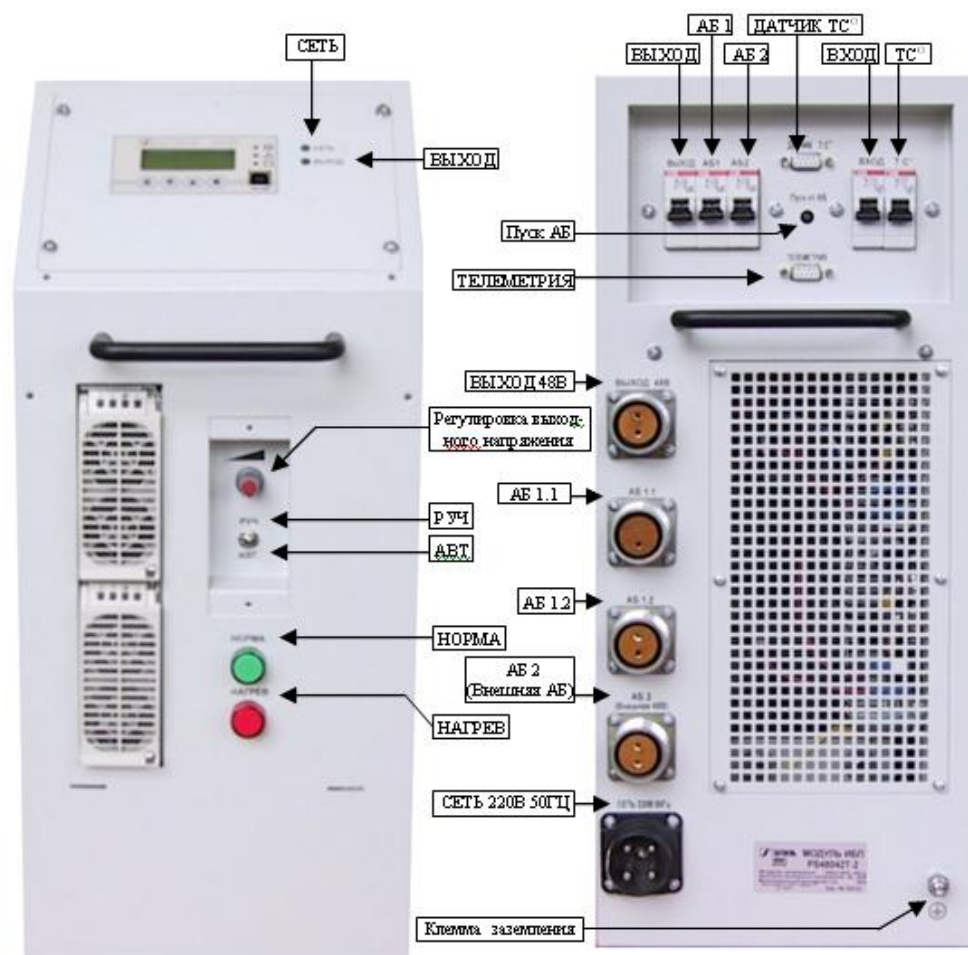
Источник бесперебойного питания постоянного тока Штиль PS48042Т-2.01
