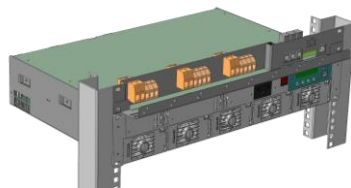
Модуль фронтального доступа DC (1U)
