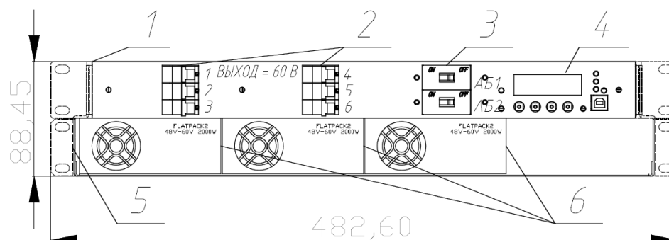
Установка питания Штиль PS60-0120-2U
