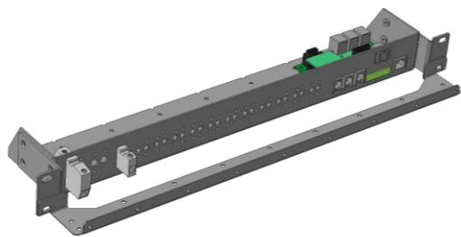
Модуль фронтального доступа DC (1U)
