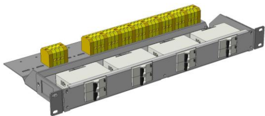
Модуль распределения Штиль MP-21-08
