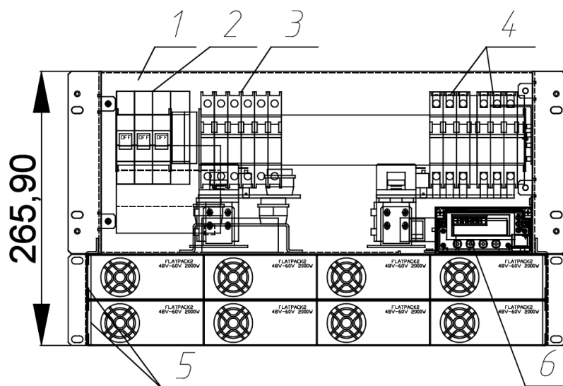
Установка питания Штиль PS60-0240
