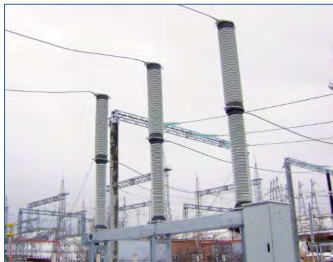
Выключатель ВГТ-1A1-220
