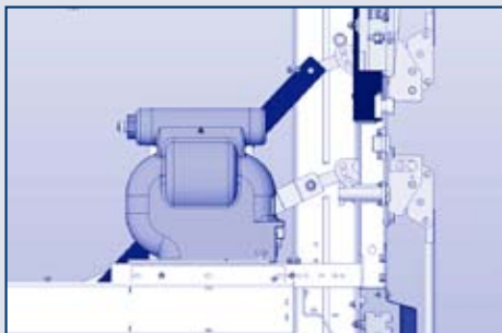
Трансформаторы напряжения в рабочем положении
