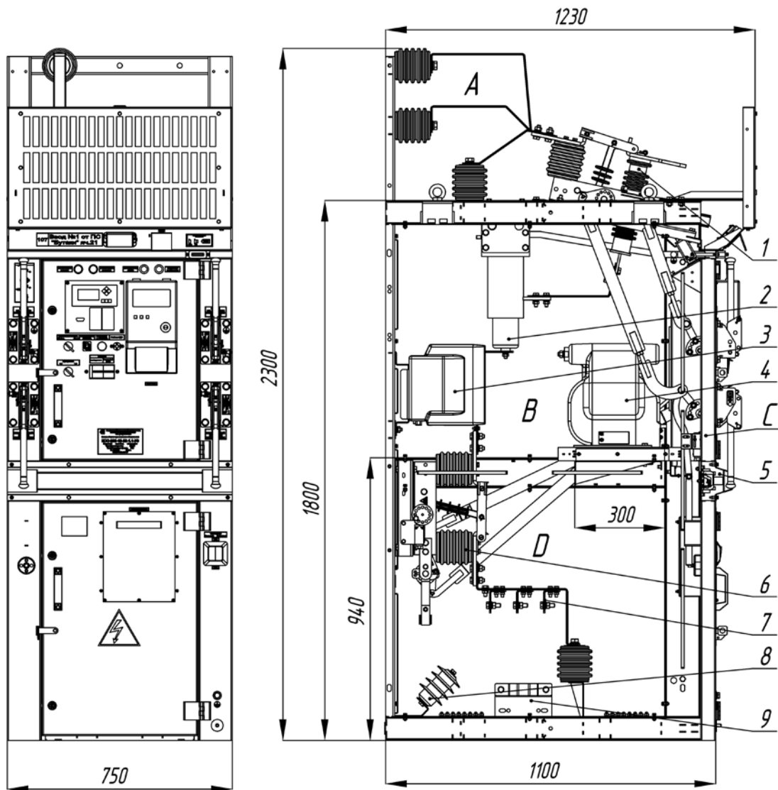
Рис. 1. Общий вид КСО-208
