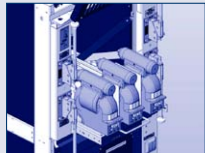
Трансформаторы напряжения в положении «выкачено»
