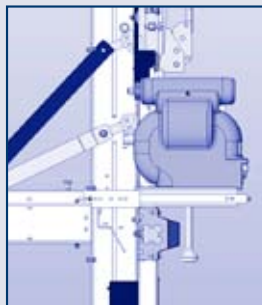
Трансформаторы напряжения в положении «выкачено»
