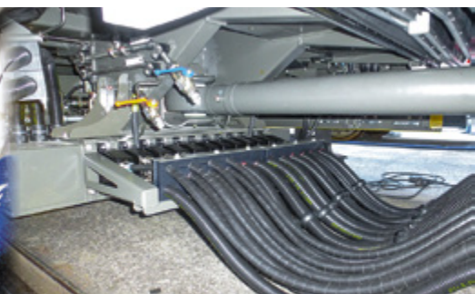
Подвагонная область
