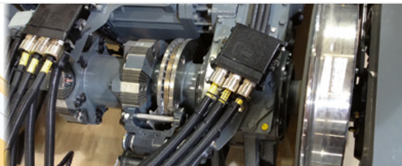
Подключение электропривода тележки
