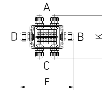
Расположение КВ и клемм
