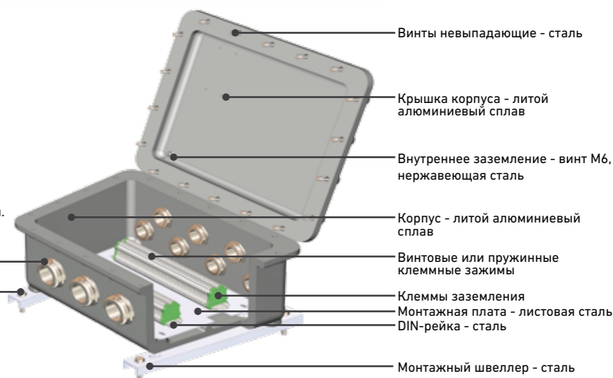
Максимальное количество кабельных вводов (КВ) производства LT, устанавливаемых на каждую сторону коробки
