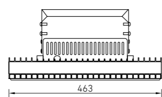
Габарит корпуса II
