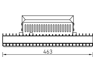
Габарит корпуса III
