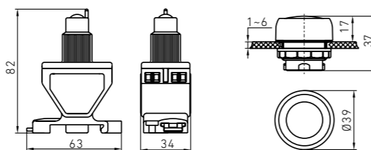
Габаритные размеры индикатора с кнопкой
