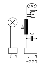
Подвод питания для рабочей и аварийной ламп. Схема подключения
