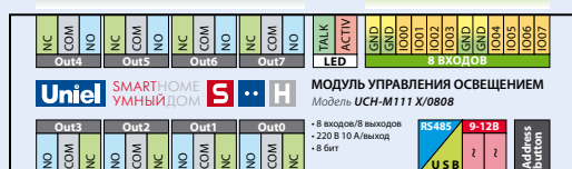
Выходы управляющих реле для подключения источников света
