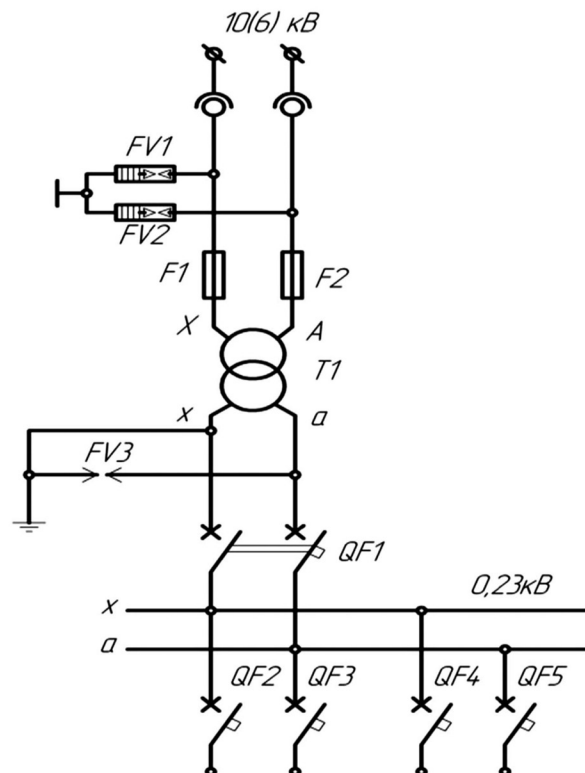
СХЕМА ЭЛЕКТРИЧЕСКАЯ ПРИНЦИПАЛЬНАЯ
