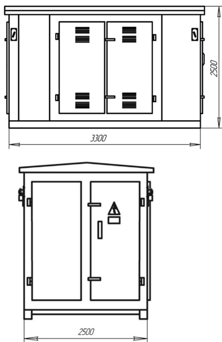
ГАБАРИТНЫЕ РАЗМЕРЫ КТПГ 25-630/10 (6) У1
