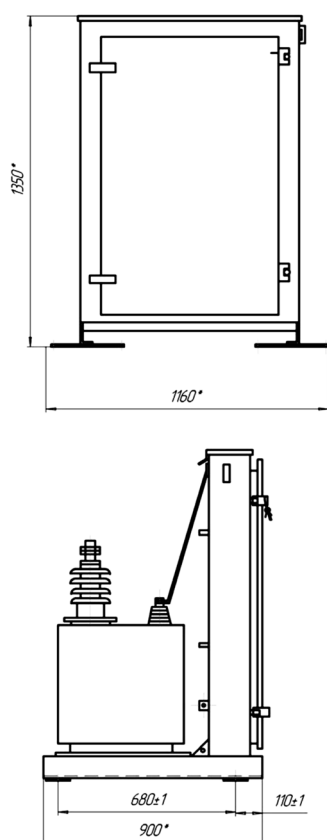
ГАБАРИТНЫЕ РАЗМЕРЫ
