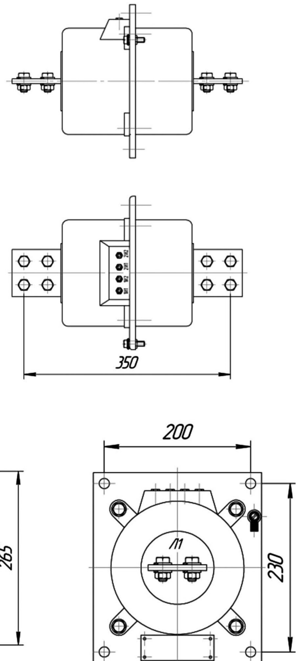
ТРАНСФОРМАТОР ТОКА ТИПА ТПОЛ-10 (800-1500/5А)
