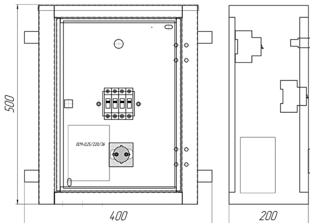
ОБЩИЙ ВИД И ГАБАРИТНЫЕ РАЗМЕРЫ
