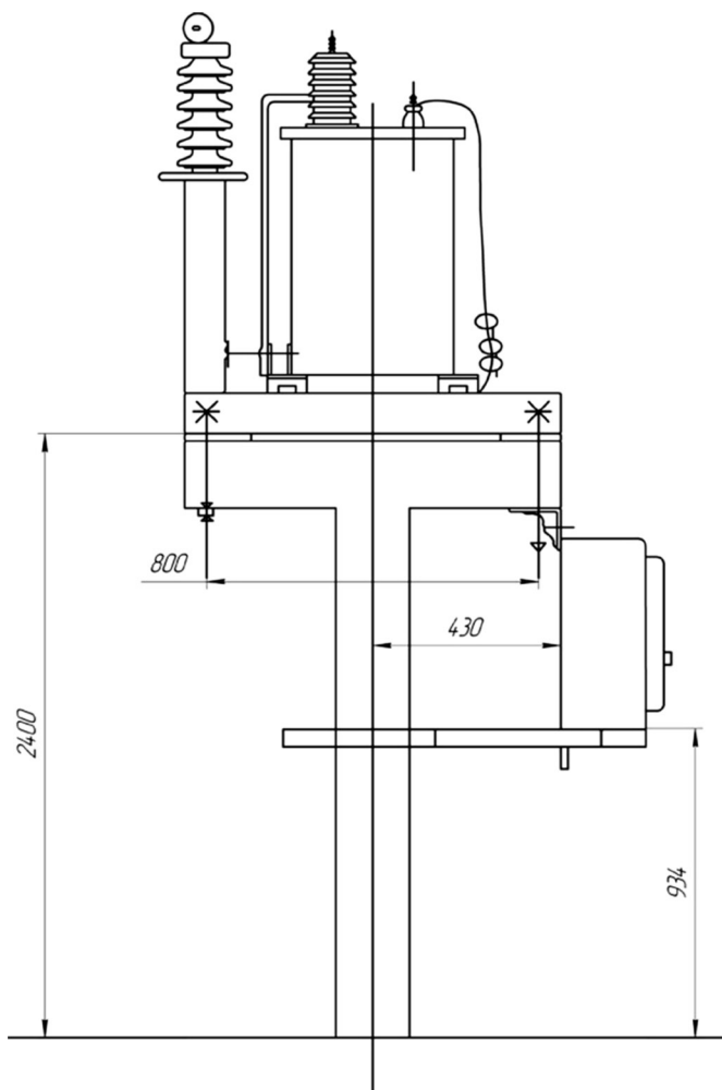
ГАБАРИТНЫЕ РАЗМЕРЫ
