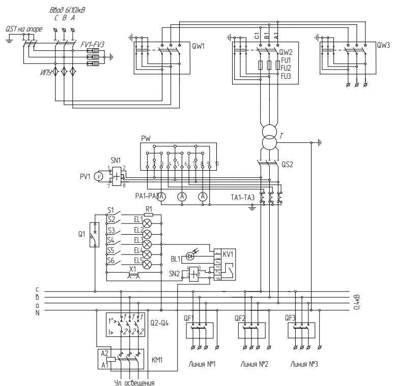
СХЕМА ЭЛЕКТРИЧЕСКАЯ ПРИНЦИПАЛЬНАЯ
