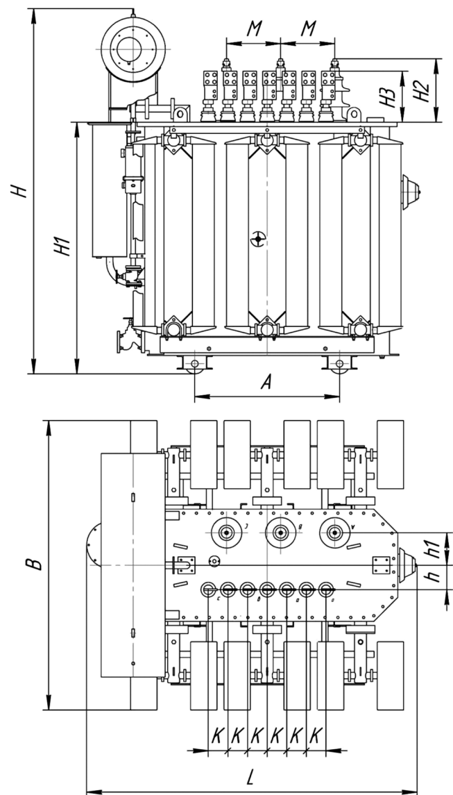
ГАБАРИТНЫЕ РАЗМЕРЫ ТРАНСФОРМАТОРА ТМ2500/35/0,4КВ
