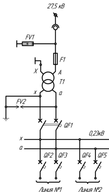
СХЕМА ЭЛЕКТРИЧЕСКАЯ ПРИНЦИПАЛЬНАЯ
