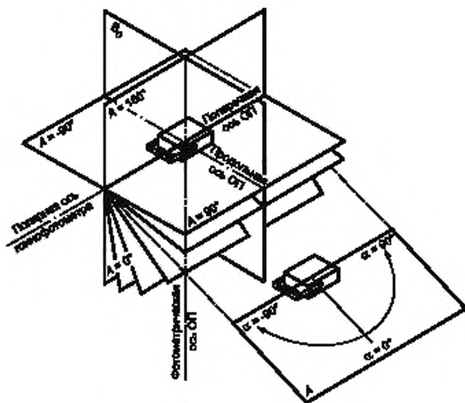
а – системы фотометрирования A, α
