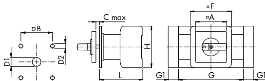
Lochbild Frontschild
