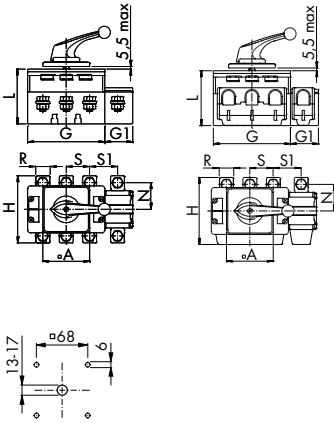
Fronteinbau 4-Loch-Befestigung
