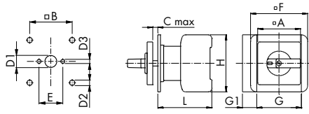
Lochbild Frontschild
