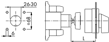
Frontschild 88 x 88: KG125-KG317
