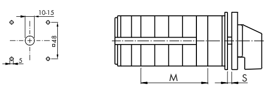
V110, V115, V130, V135, 4-Loch-Befestigung (Baugröße S1)
