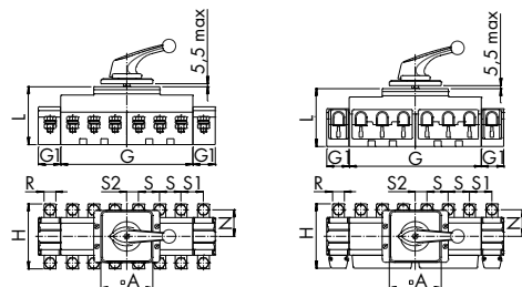
Fronteinbau 4-Loch-Befestigung
