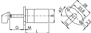
E93, E94 Maß L auf Seite 117
