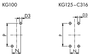
Lochbild Boden (Befestigung auf Normschiene bis KG100)
