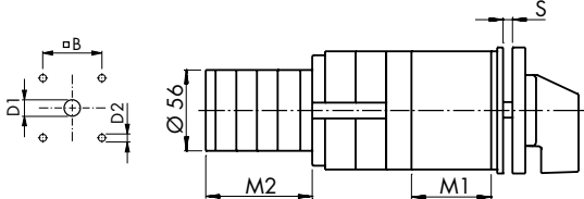
V120, 4-Loch-Befestigung (Baugröße S1) V110, V120, V130, 4-Loch-Befestigung (Baugröße S2 + S3)
