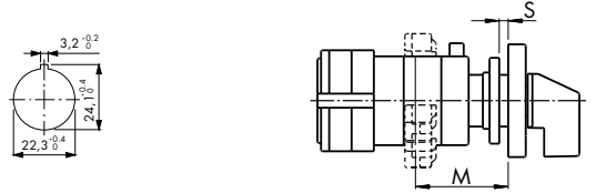
V110A–V135A, Zentralbefestigung (Baugröße S0)
