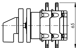
CH...-4 (Stecker gerade 2 x 2,8 oder 1 x 6,35)
