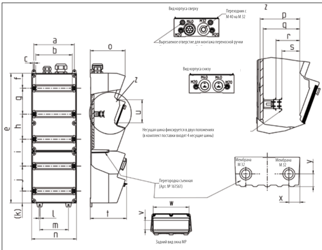
Чертеж 1 MB 571-5
