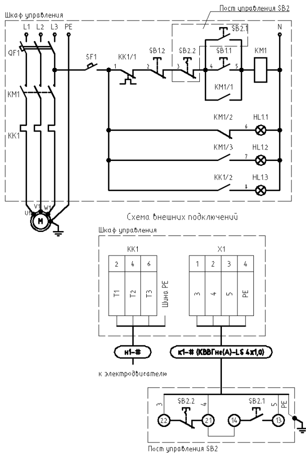
Принципиальная схема управления электродвигателем
