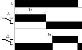
Диаграмма работы пускового реле (звезда-треугольник)
