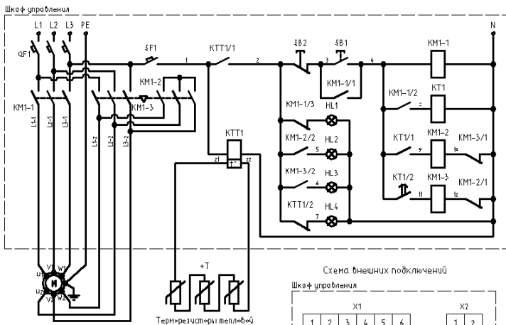
Терморезисторы тепловой защиты двигателя
