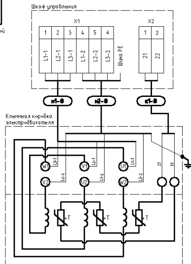
Схема внешних подключений
