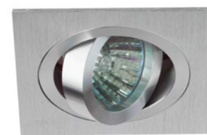
KL57 A-SL серебро ↔ 120x120мм ⌀ 105 мм ↓ 20 мм → 220V
