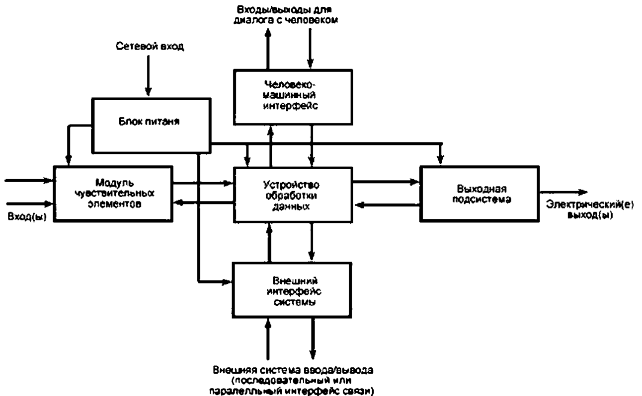
Рисунок А.1 – Модель измерительного устройства
