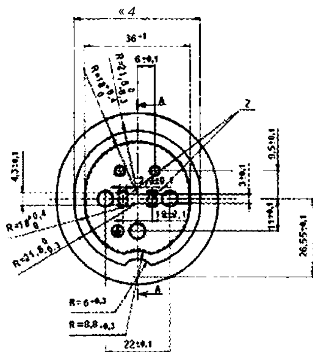
Расположение штырей ( )
