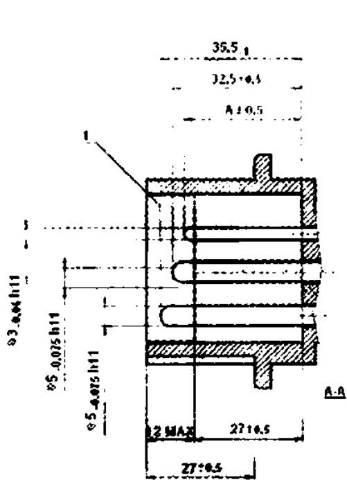
Конец штырей
