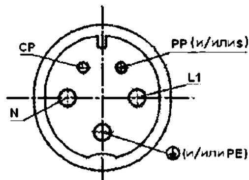
Расположение штырей ( )
