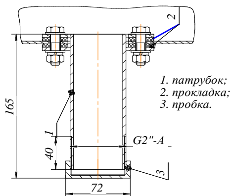
Д-Д (1:2,5) \ominus 90^\circ Рабочее положение патрубка
