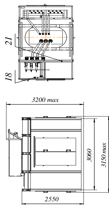
Рисунок А.2 - Транспортное положение
