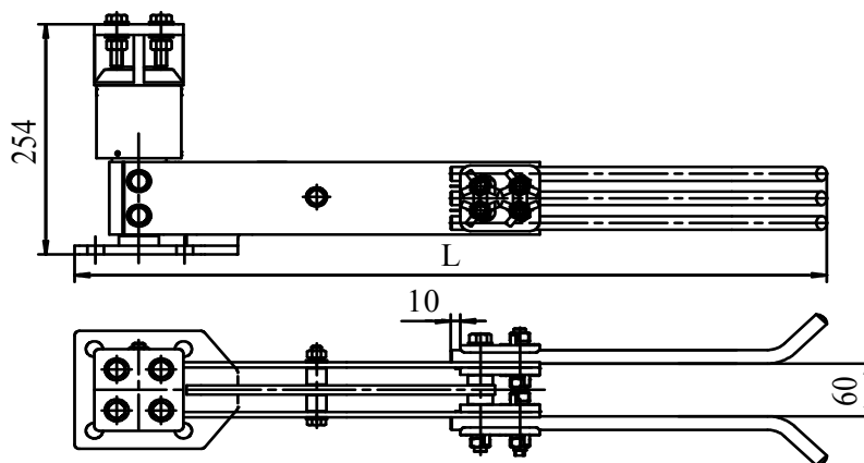
Рисунок 20 – Нож контактный для РН(П)(С)К СЭЩ-110/2000
