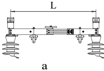
Главные ножи РН(П) СК на 2000 А
