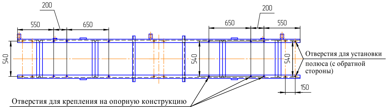
Рисунок 5 – Разметка отверстий на общей раме для крепления ее на опорную конструкцию
