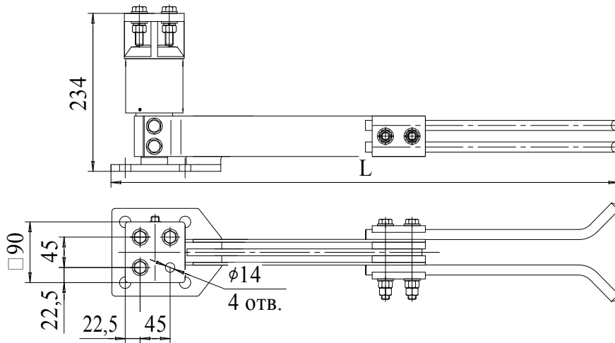
Рисунок 18 – Нож контактный для РН(П)(С)К СЭЩ-110/1250
