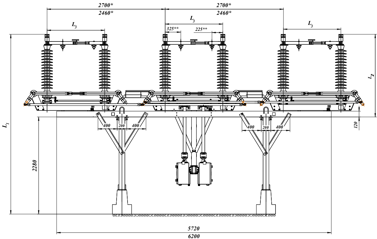
Рисунок 14 – Общий вид разъединителя РН К СЭЩ-□ - □-110/□□
