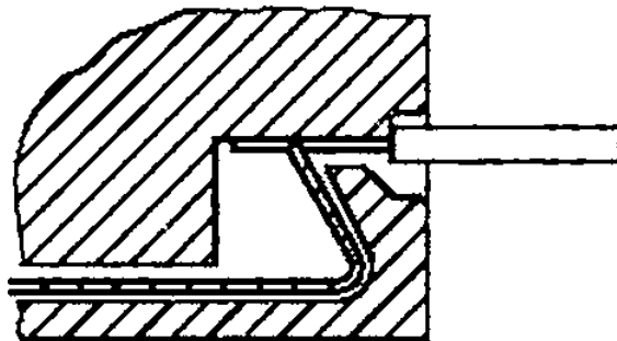
Рисунок 2 б) — Пример недопустимого для использования винтового пружинного лепесткового зажима
